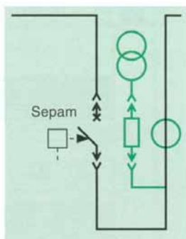
Acoplamiento cuadro BS-B (transformador de tensión opcional)
