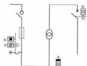
Esquema tipo R8
