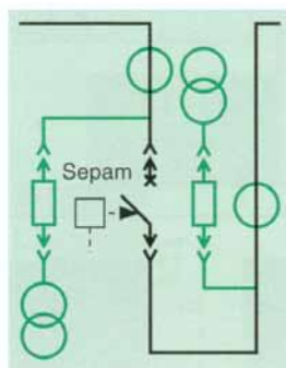
Acoplamiento cuadro BS-B (transformador de media opcional para MCset 1-2-3)
