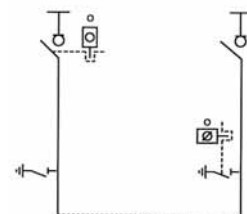
Esquema tipo R1
