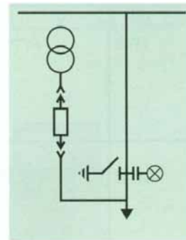
Medida y puesta a tierra del juego de barras BB-V
