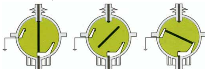
aparato cerrado
