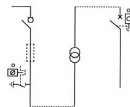
Esquema tipo R6
