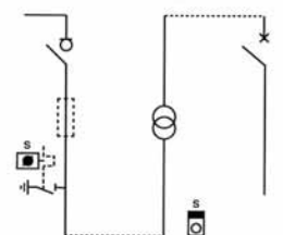
Esquema tipo R7
