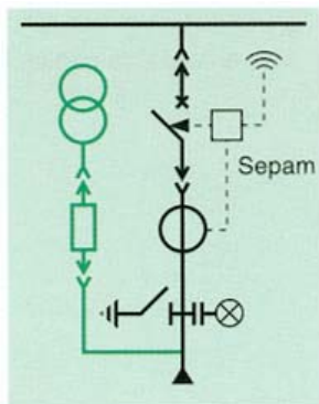
Entrada LI-B, TI-B, GI-B (transformador de tensión opcional)
