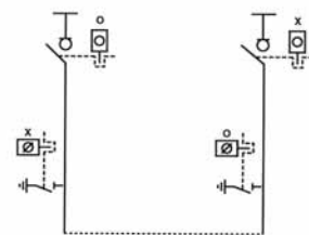
Esquema tipo R2
