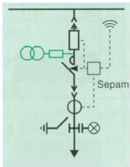
Salida contactor-fusibles MF-C, CB-C (transformador de tensión opcional)
